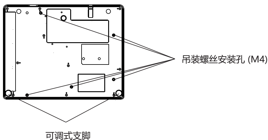
吊装螺丝安装孔及可调节式支脚的位置
